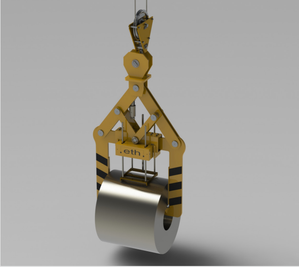
Mekanik Yatay Bobin Taşıma Ataşmanı
