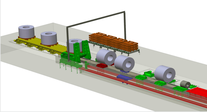
Bobin Paketleme ve Devirme İstasyonu
