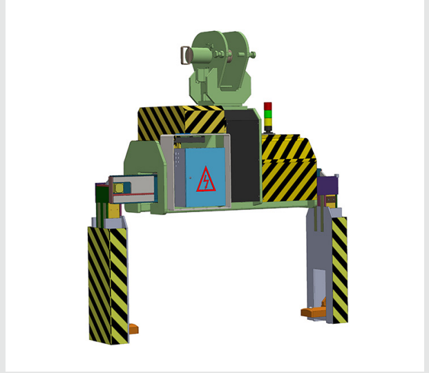
Tırnakları Açılıp Kapanır Yatay Bobin Taşıma Ataşmanı
